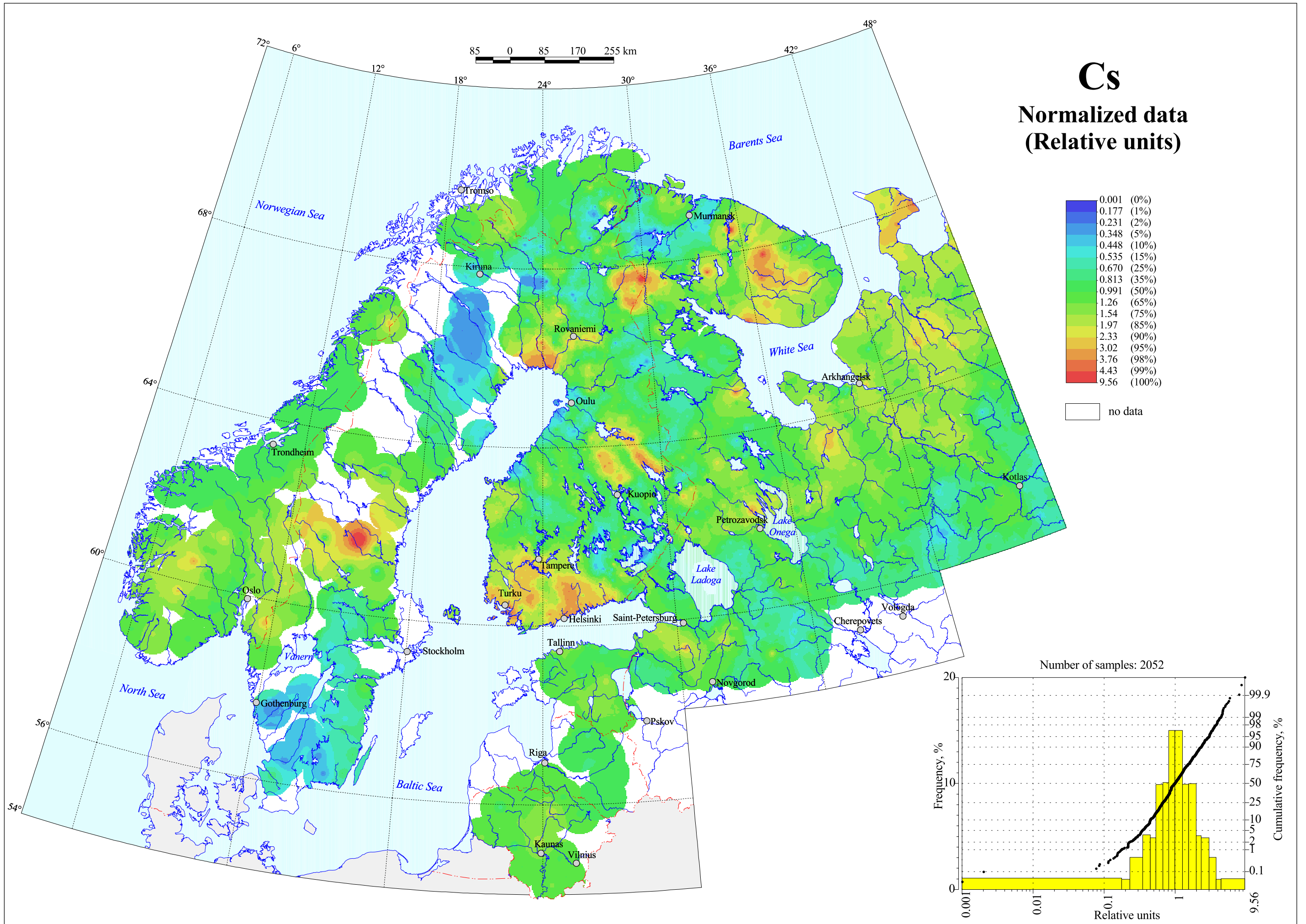
Cesium in Stream Sediment
